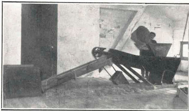
Una máquina lavadora, funcionando.
