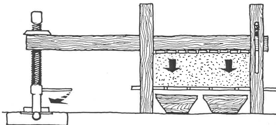
AURREKO GIZALDIEK ERABILTZEN ZUTEN HABE-LUZEKO TOLAREA
